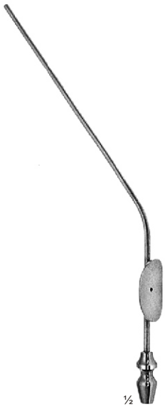
BARNES 21-159-16 16 cm, 6¼"
